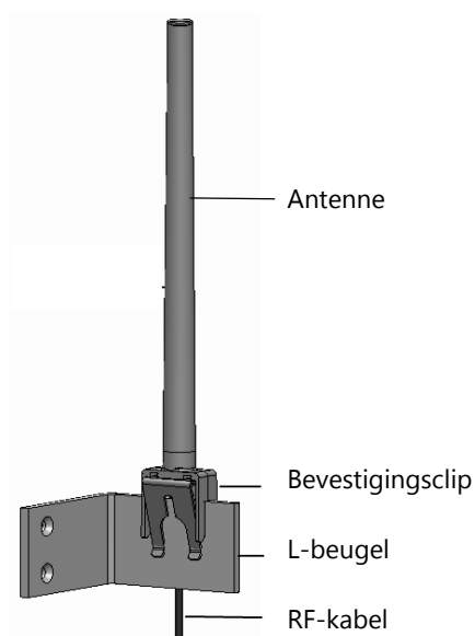
Afbeelding 3. Antenne die aan de beugel is bevestigd
